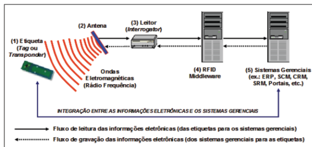
Figura 1: Esquemática do sistema básico de RFID
